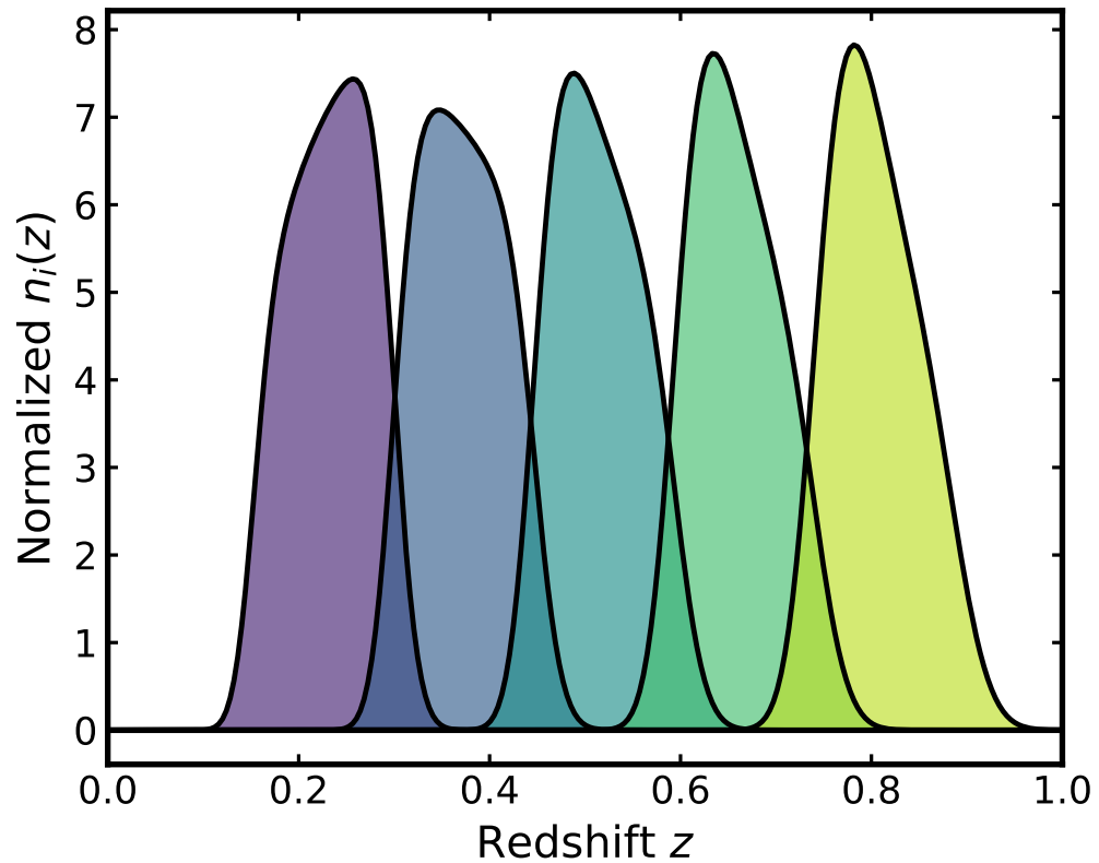
DES lens bins
