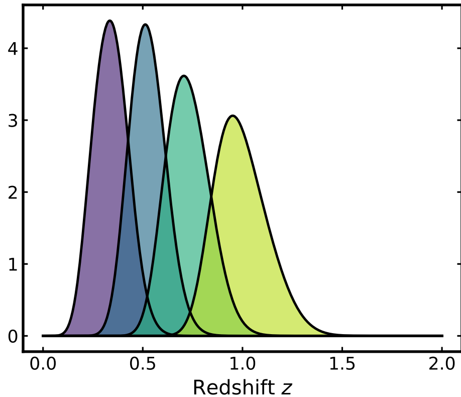
DES source bins
