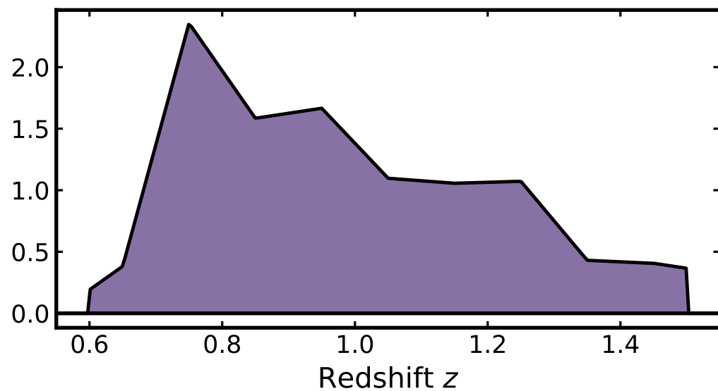
DESI ELG: one bin
