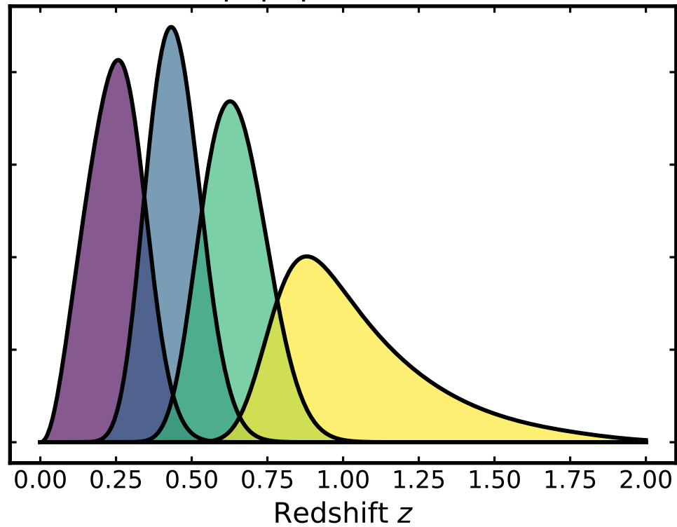
Equipopulated bins
