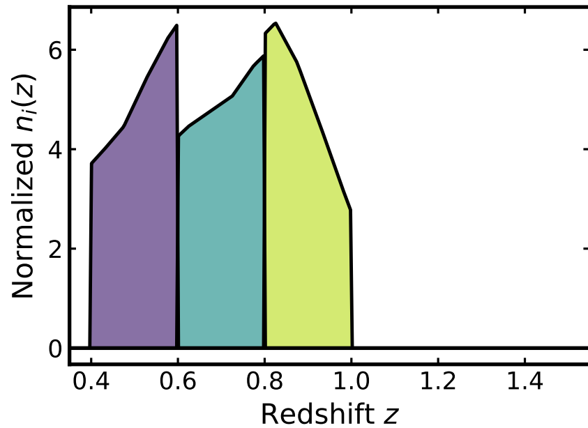
DESI LRG bins
