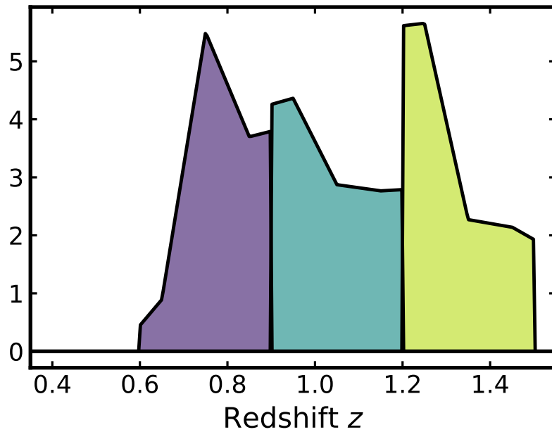
DESI ELG bins
