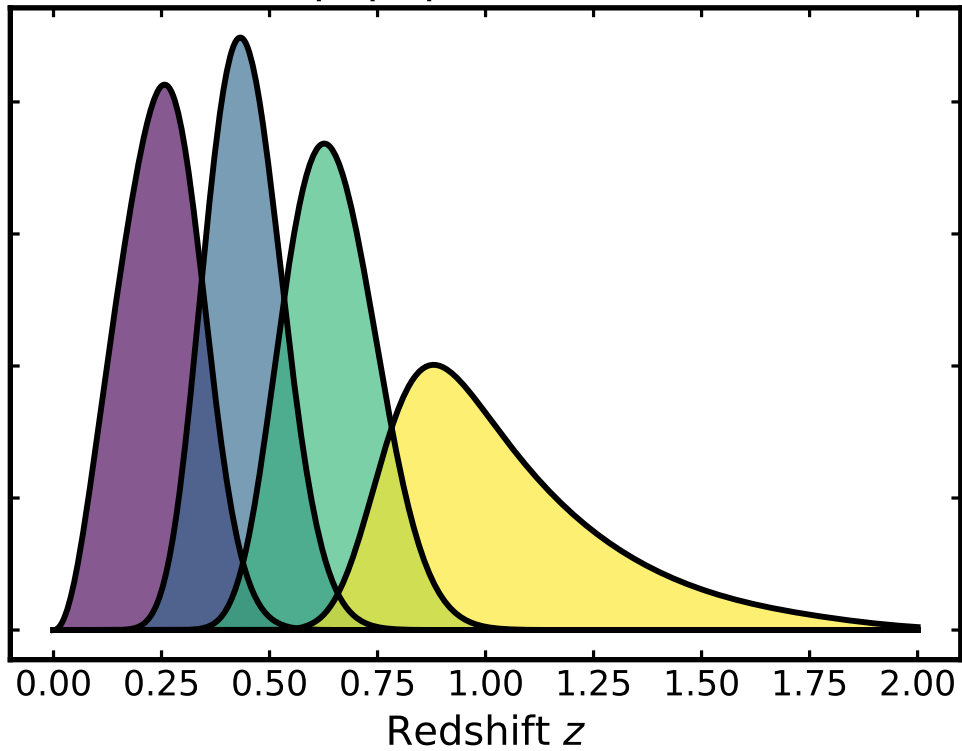
Equipopulated bins
