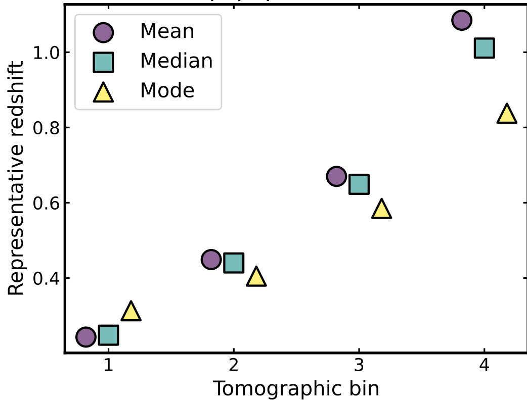
Equipopulated bins
