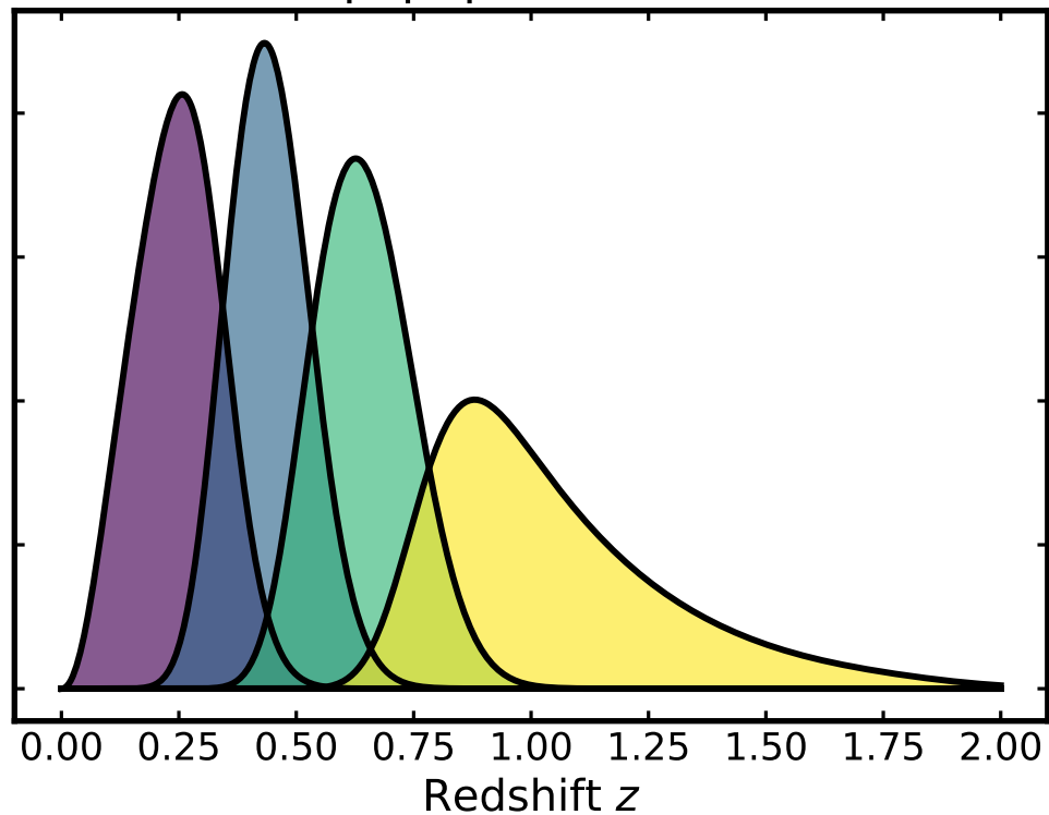
Equipopulated bins
